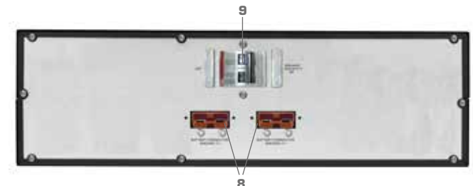
Module d'autonomie E7 One 10k RT (3U)
